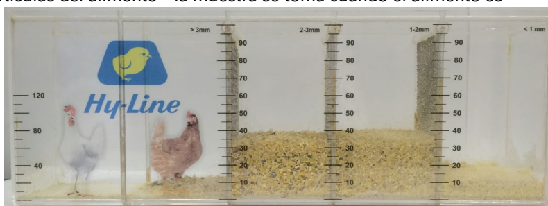
Tamizador Hy-Line
